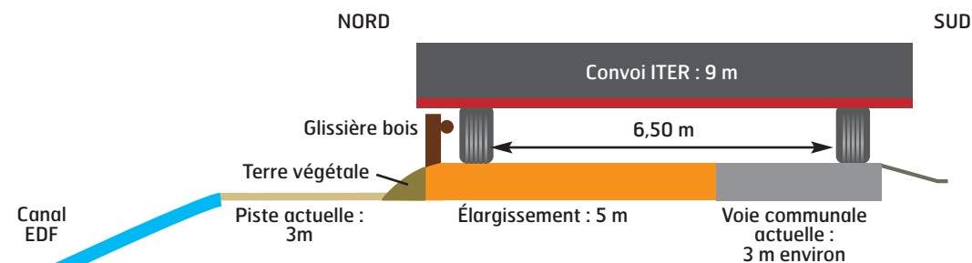
L'élargissement de la voie côté canal
